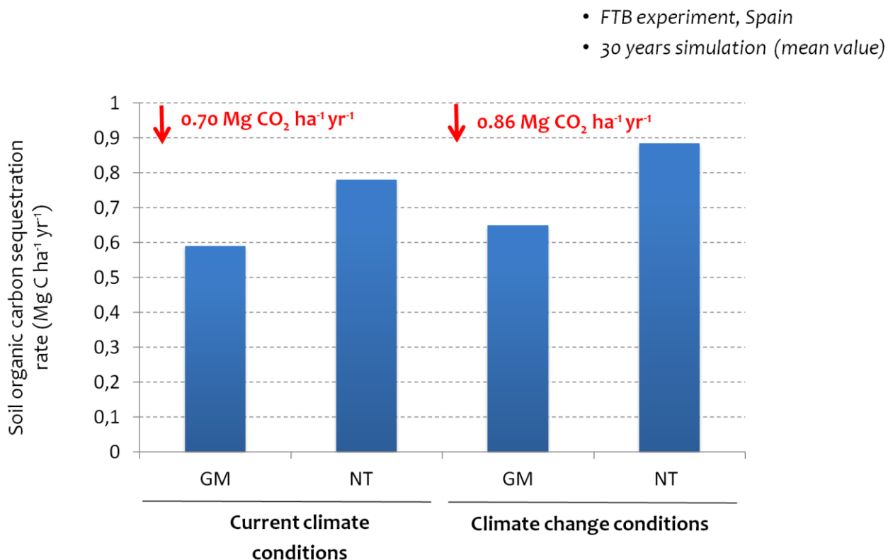
2.attēls. Simulācijas dati CO 2 emisiju mazinājumam Spānijā, izmantojot projektā iegūtos rezultātus
